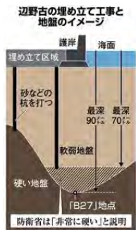
地盤のイメージ
